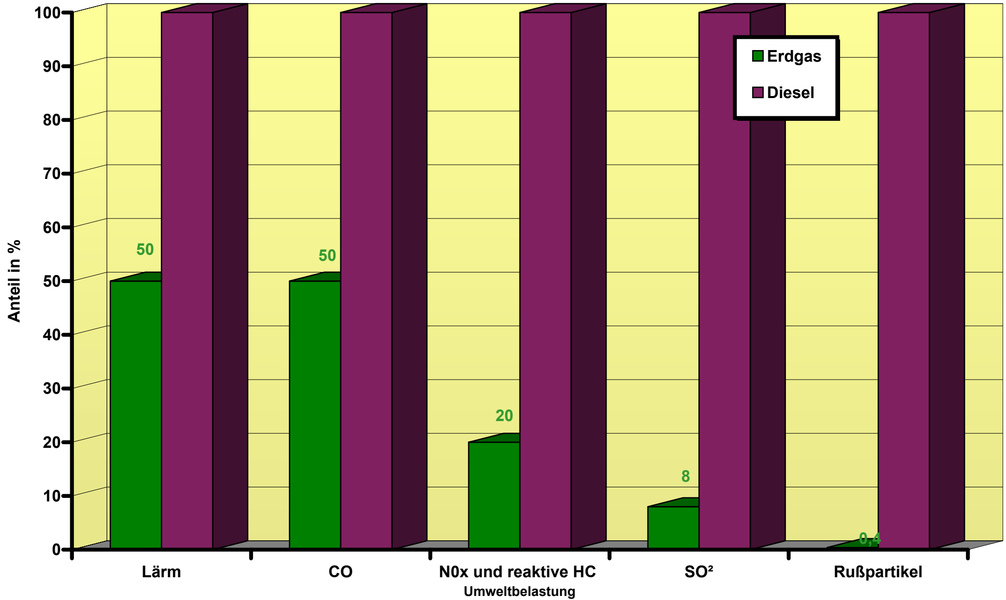
Emissionsvorteile von Erdgasnutzfahrzeugen im Vergleich zum Diesel (Quelle: verschiedene Quellen, u.a. Umweltbundesamt und MAN)
